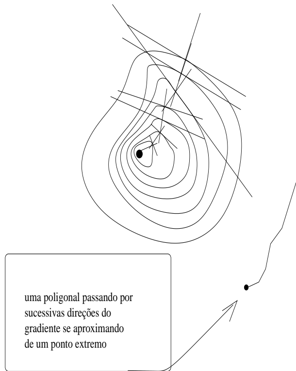
Figura 2: Uma poligonal em direção a um extremo
