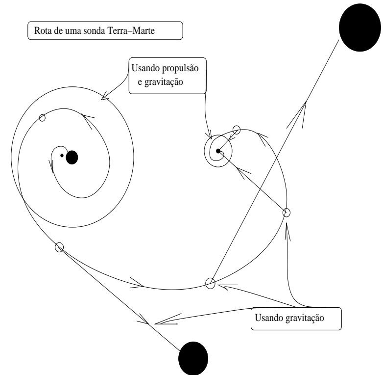
Figura 3: rota Terra-Marte de um navio espacial
