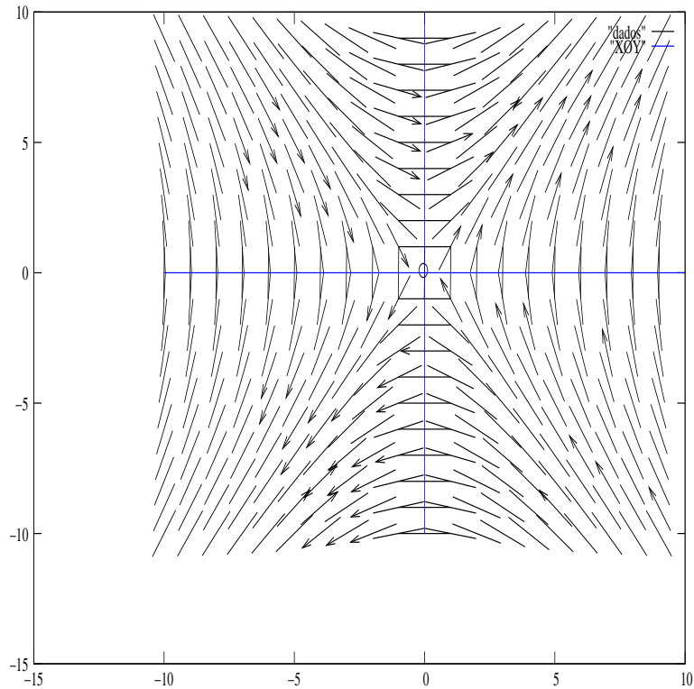
Figura 4: Campo vetorial - modelagem de uma equação diferencial
