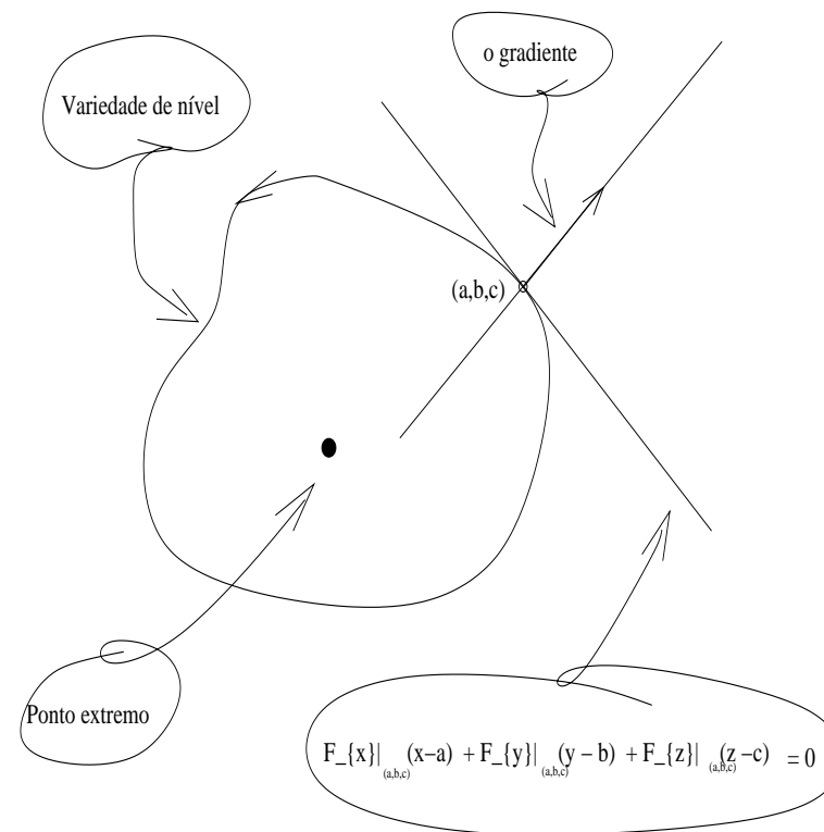
Figura 1: Um caminho para o MinMax de F
