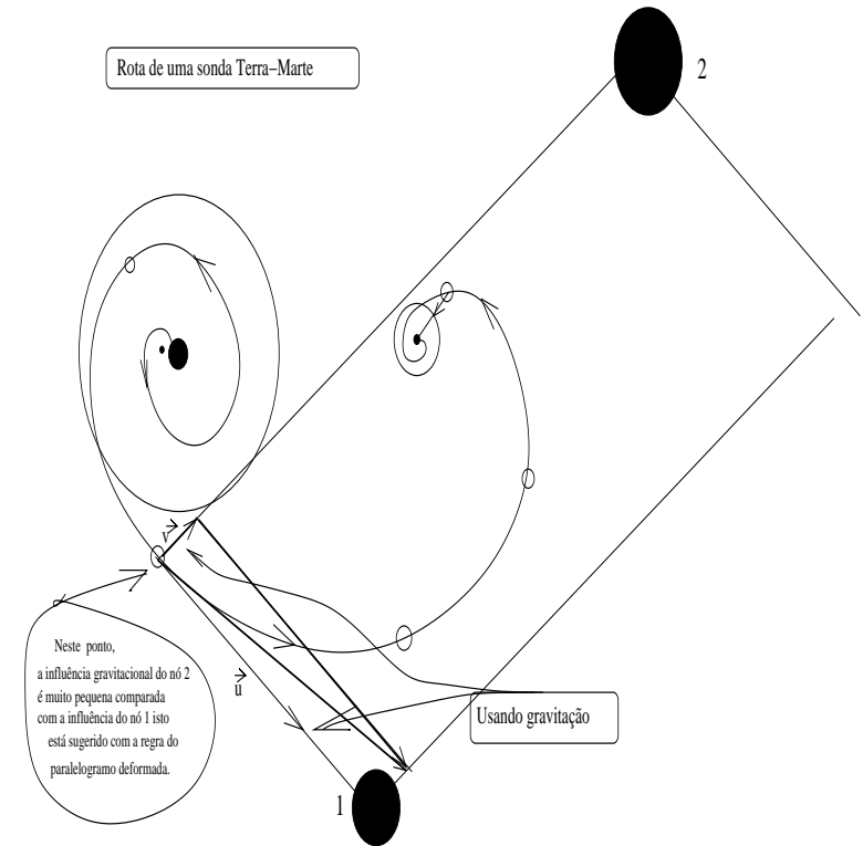
Figura 6: A derivada direcional
